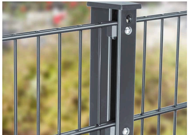
Zaunpfosten Typ XAA mit Doppelstabgitter, Anthrazit RAL 7016 · Foto: deutsche zauntechnik
